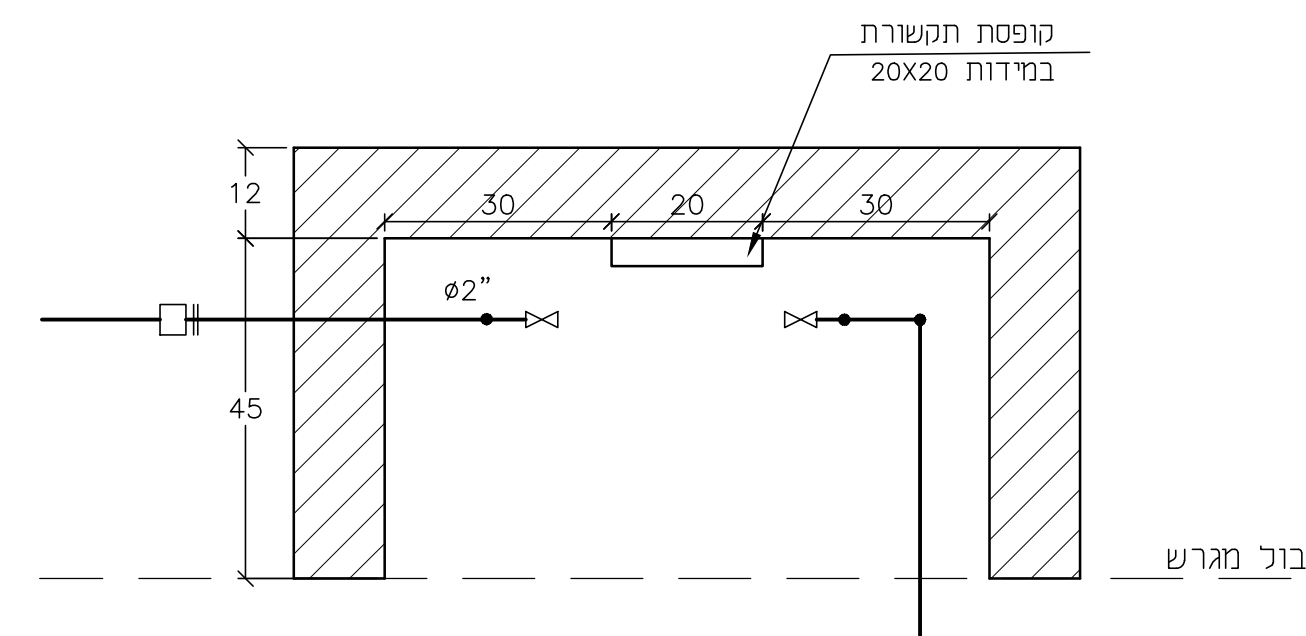
פרט מסי' 2 מיכלול מגוף חוצץ
