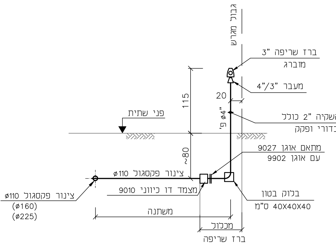
פרט מסי' 1 הרכבת ברז שריפה (הידרוט)
