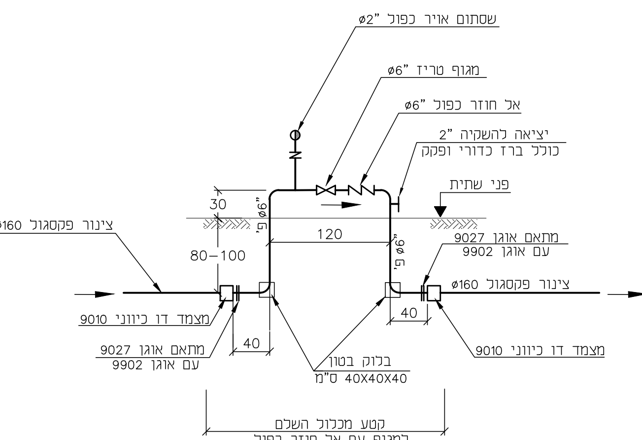
פרט מסי' 4 מיכלול מגוף חוצץ עם אל חוזר כפול
