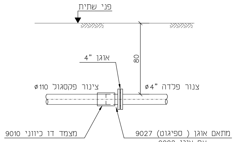
פרט חיבור לקו פלדה קיים
