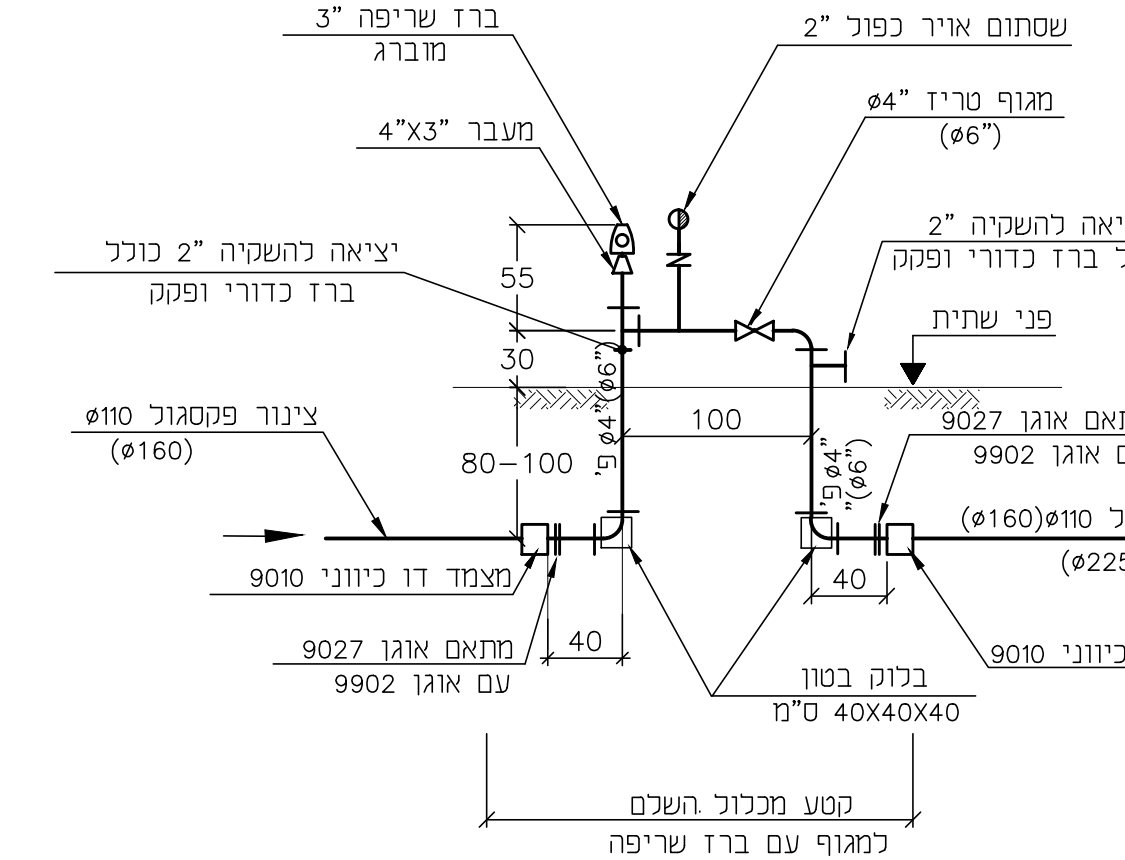
פרט מסי' 3 מיכלול מגוף חוצץ עם ברז שריפה
