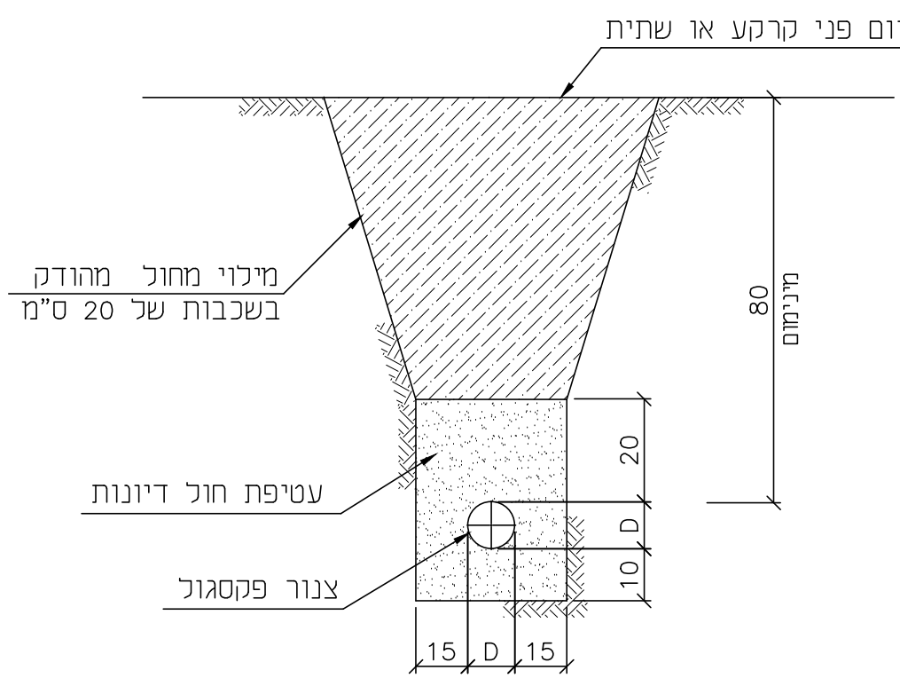
חנת צנור בתעלה כלא ק.מ.
