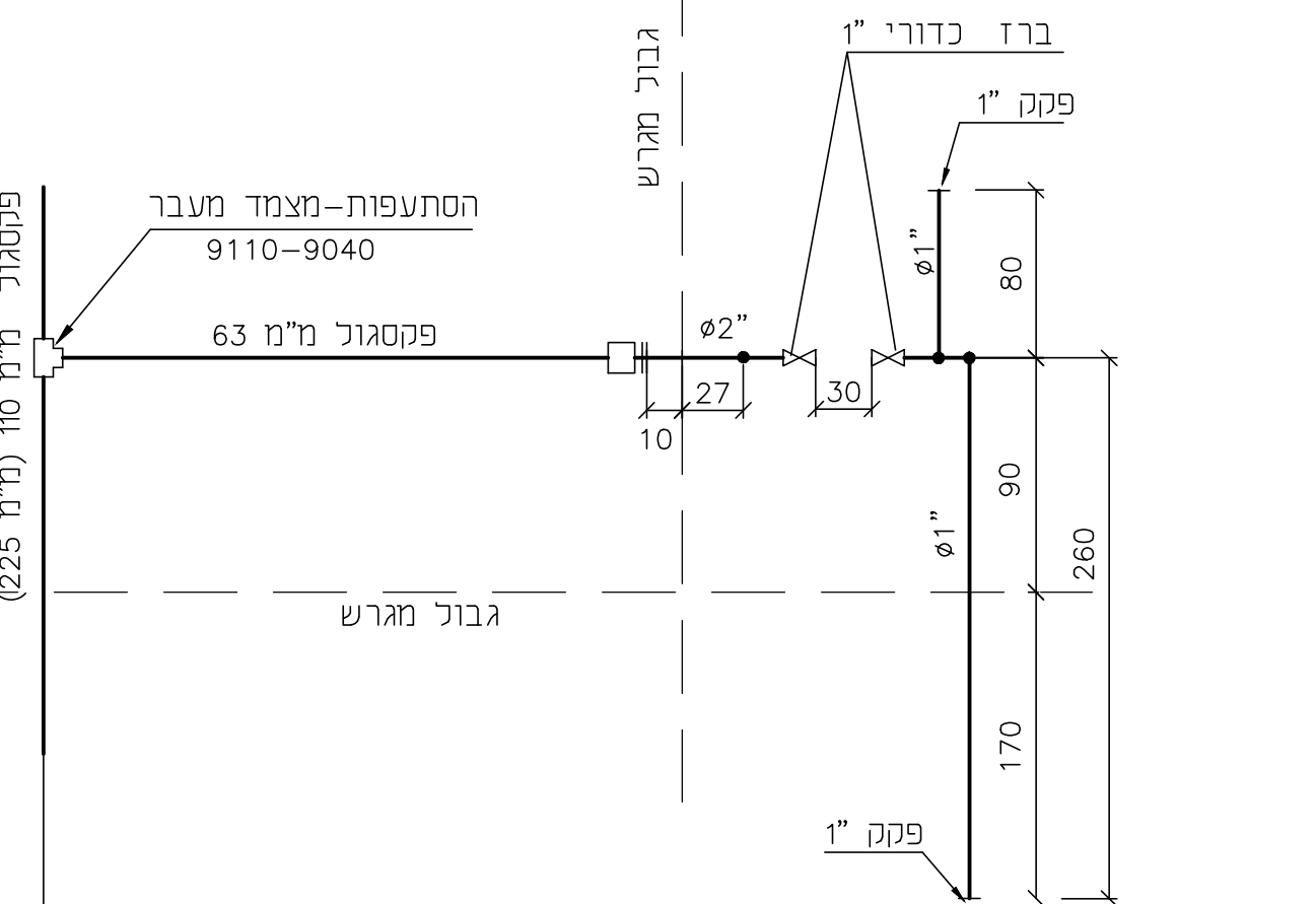
חיבור בית כפול
