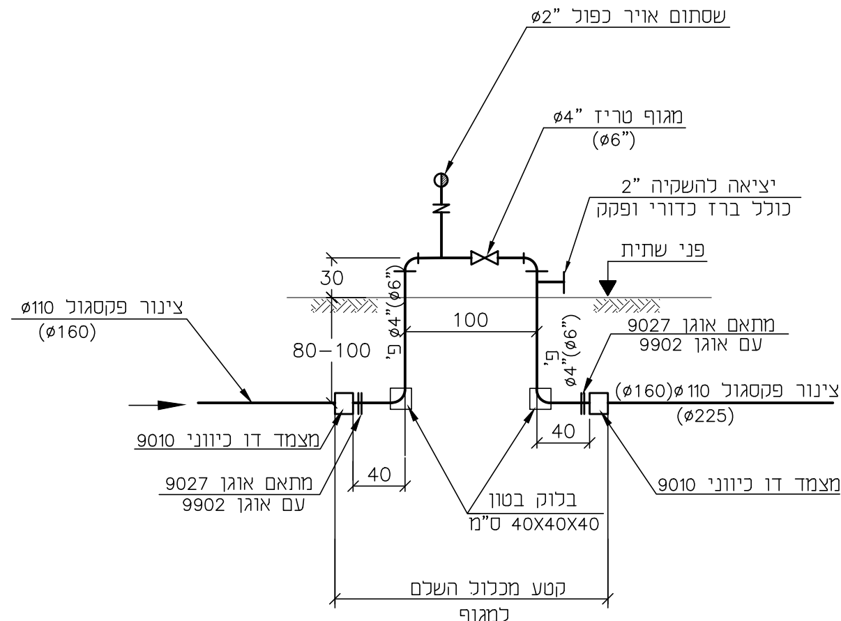
פרט מסי' 2 מיכלול מגוף חוצץ
