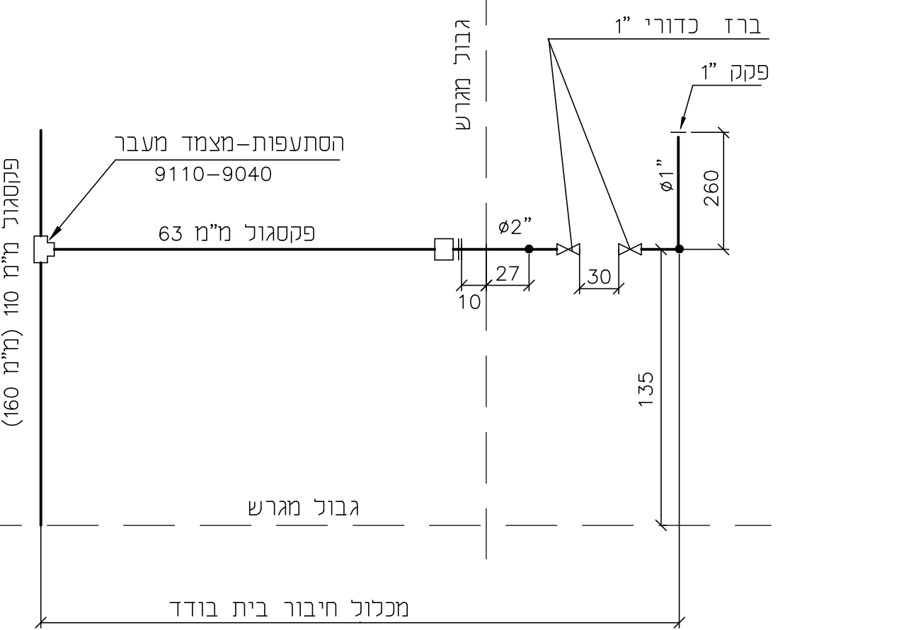
חיבור בית בודד ליציאת גינון
