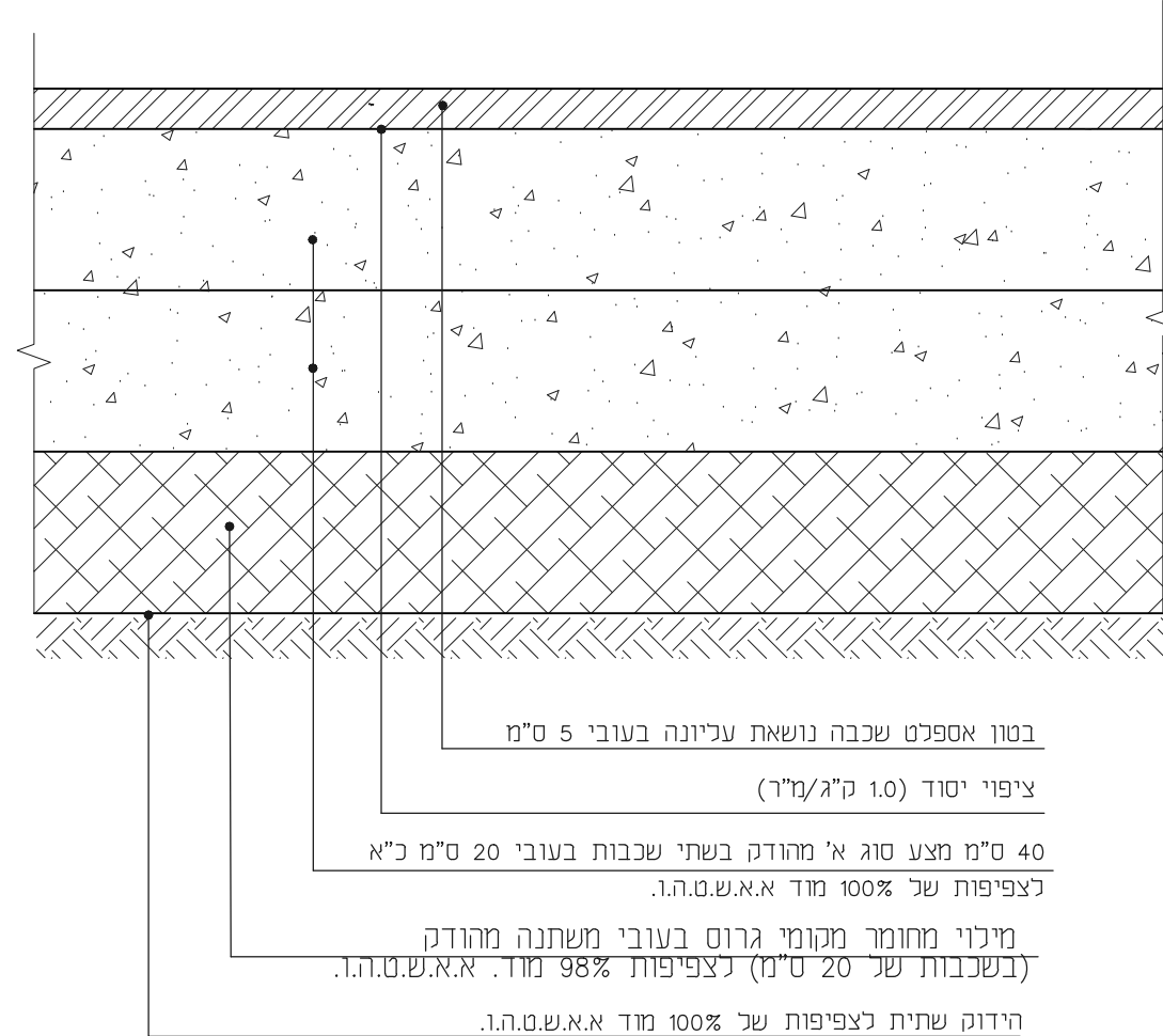
פרט מבנה דרך פטרולים במילוי
