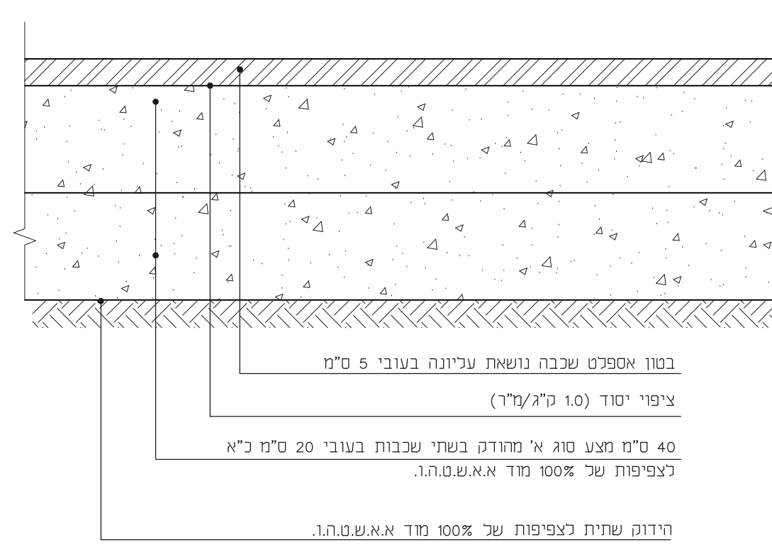
פרט מבנה דרך פטרולים בחפירה
