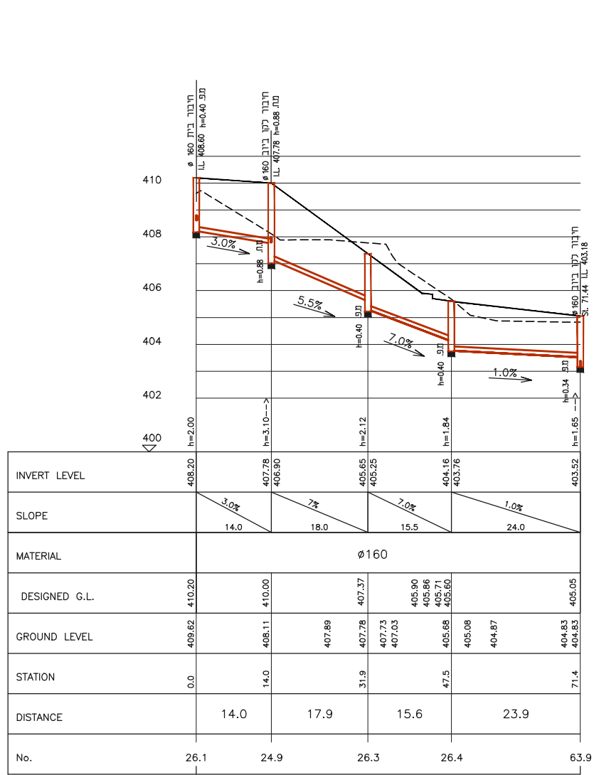
שצ"פ מגרש 728
