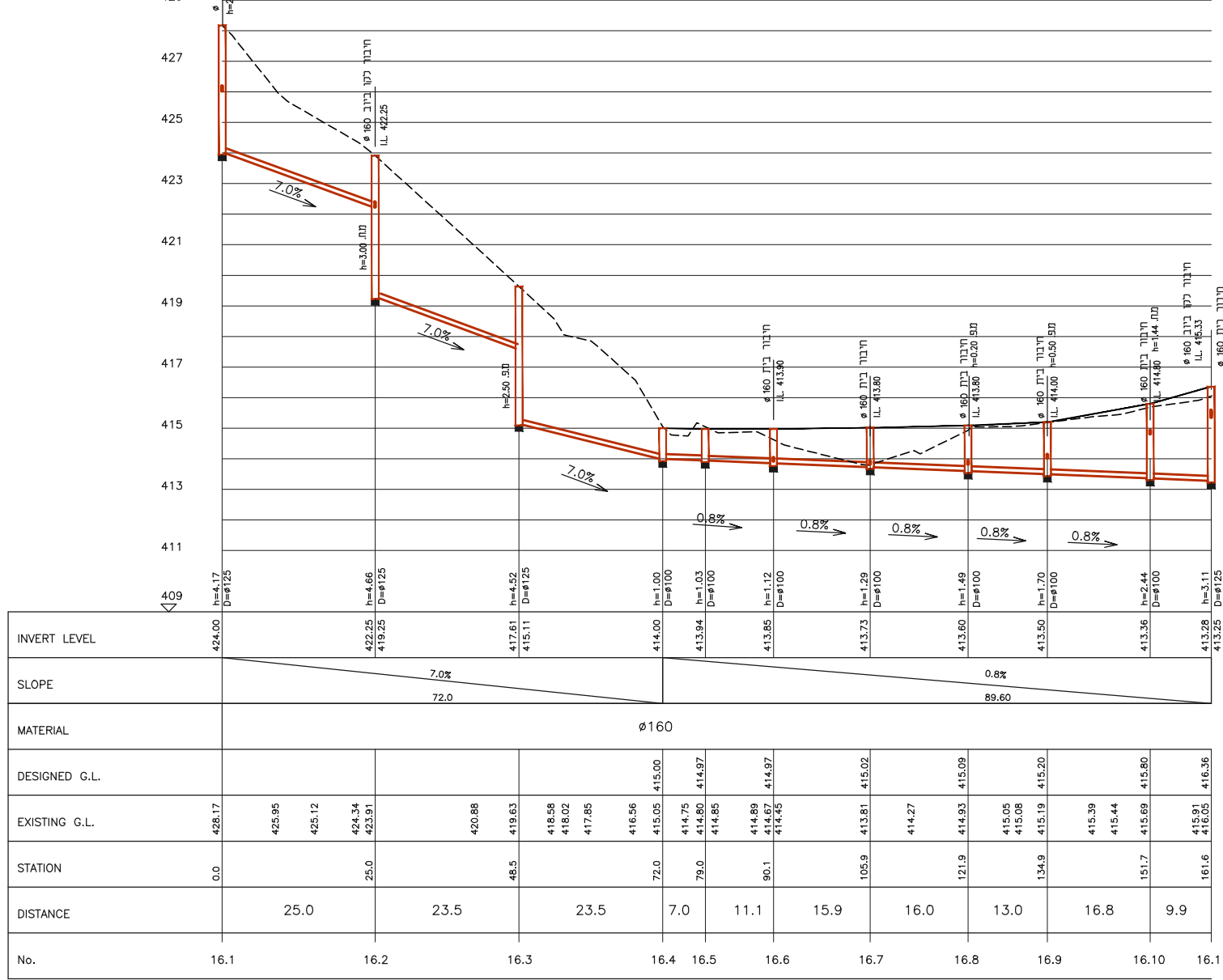
מגרשים 701, 704-707
