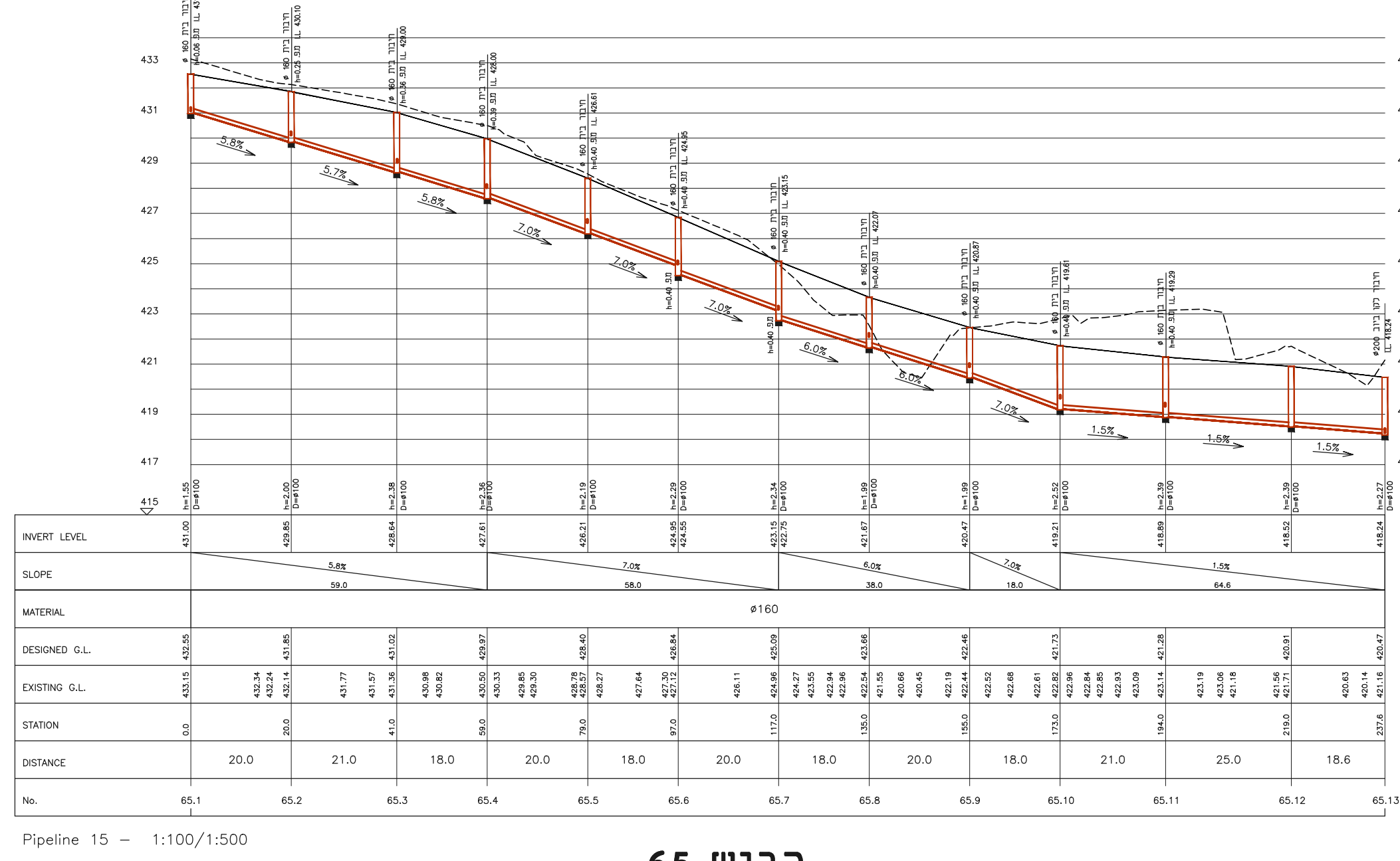
כביש 65
