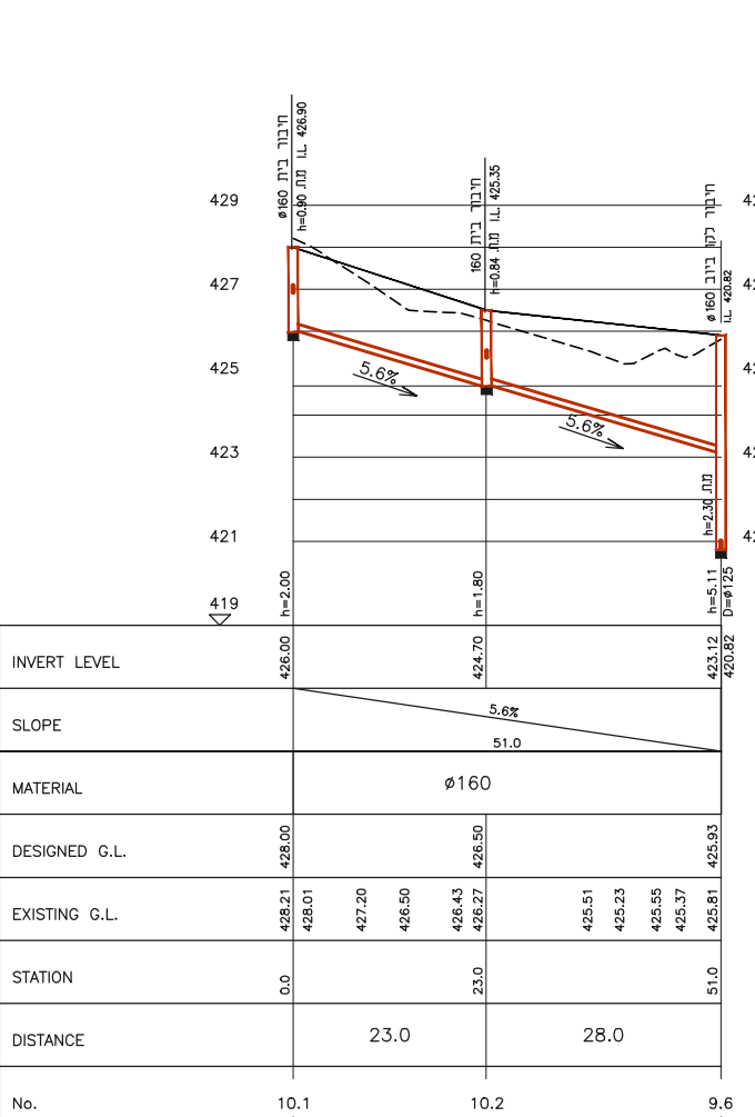
מגרשים 282-284
