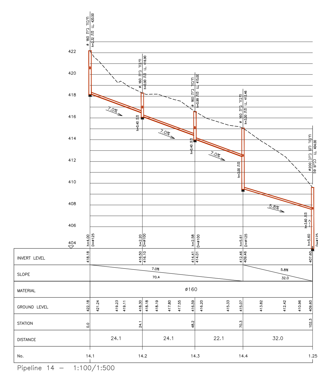
מגרשים 243-246
